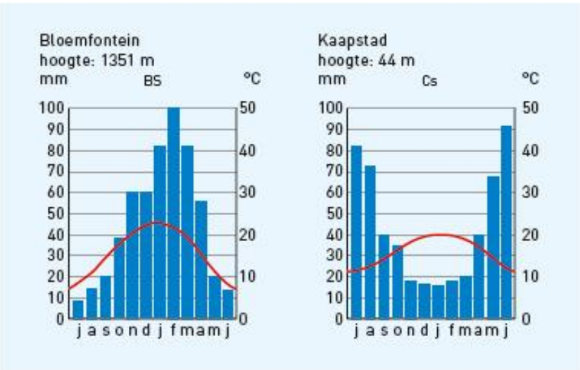
Klimaatgrafieken van Bloemfontein en Kaapstad
