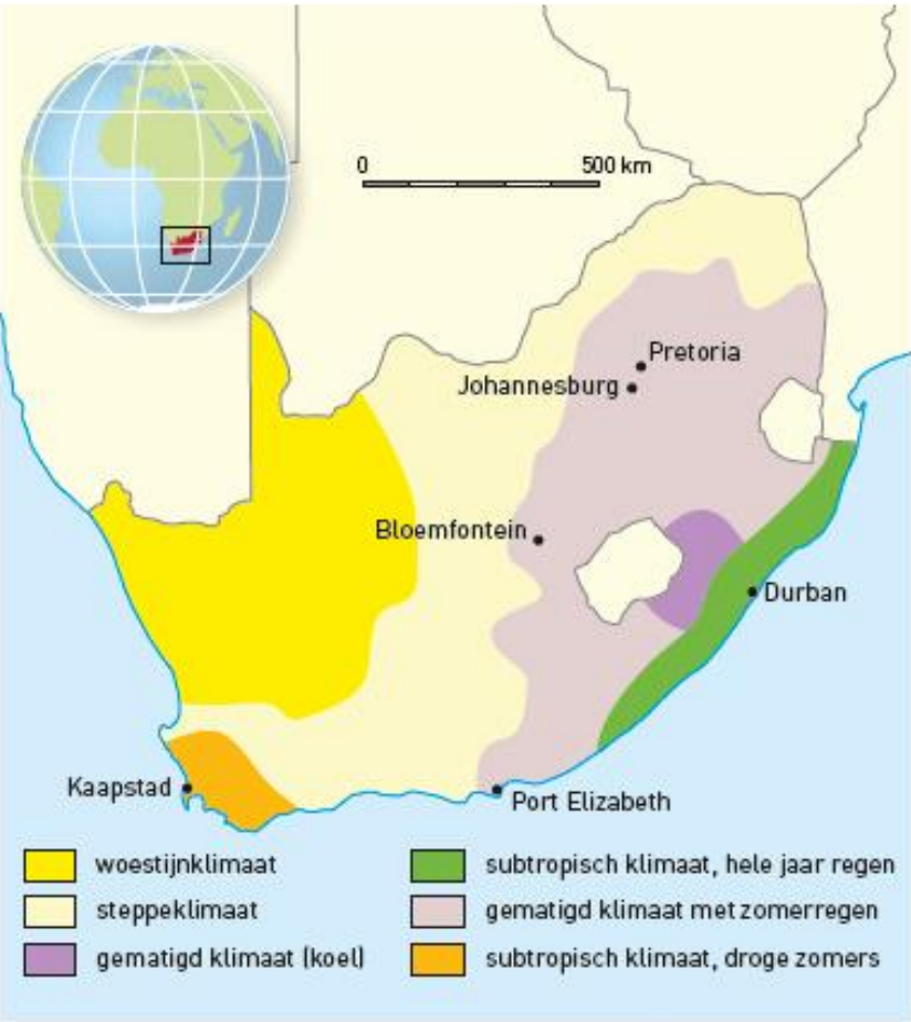
Klimaatkaart van Zuid-Afrika
