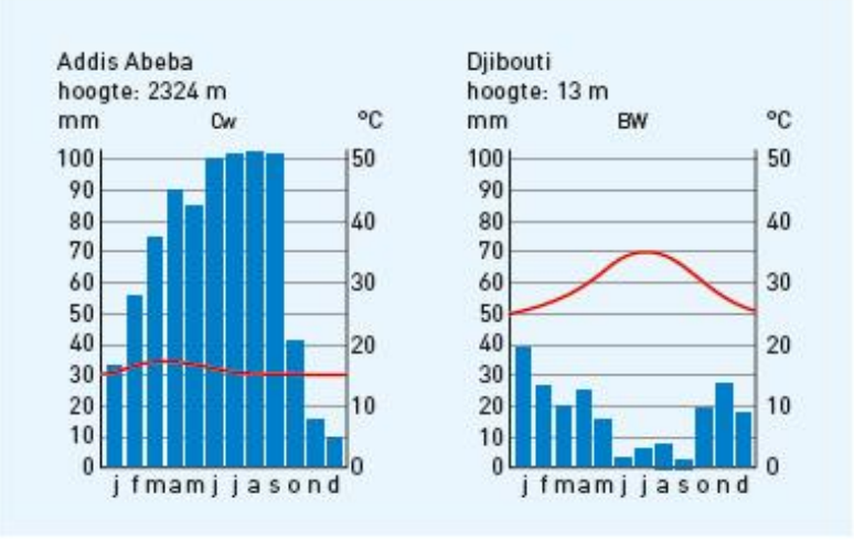
Klimaatgrafieken van Addis Abeba en Djibouti
