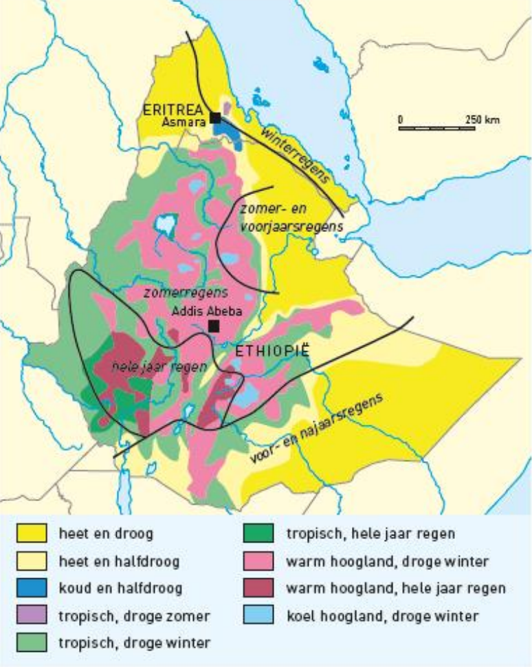
Klimaatkaart van Ethiopië
